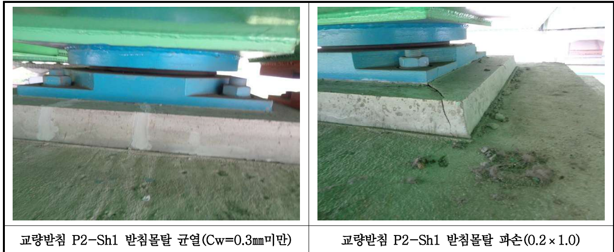
【사진 22.3.11】 교량받침 손상현황
